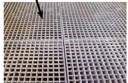
Nach der einfachen manuellen Reinigung der Roste durch Abkehren oder Bürsten ohne Stillstandszeiten ist die Kabine wieder funktionsbereit.
